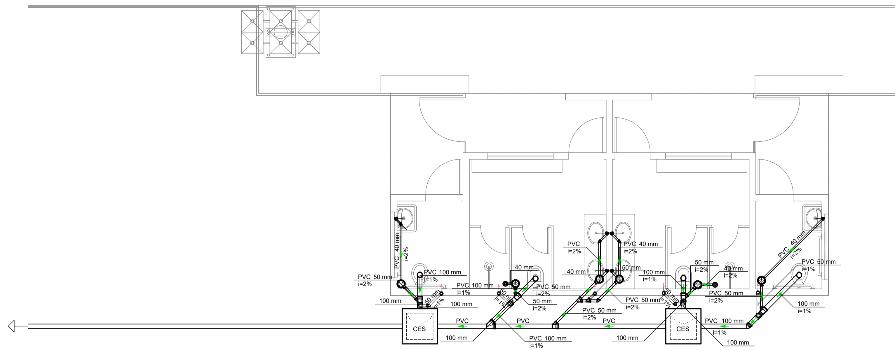
1 PLANTA BAIXA ESCALA 1:50
