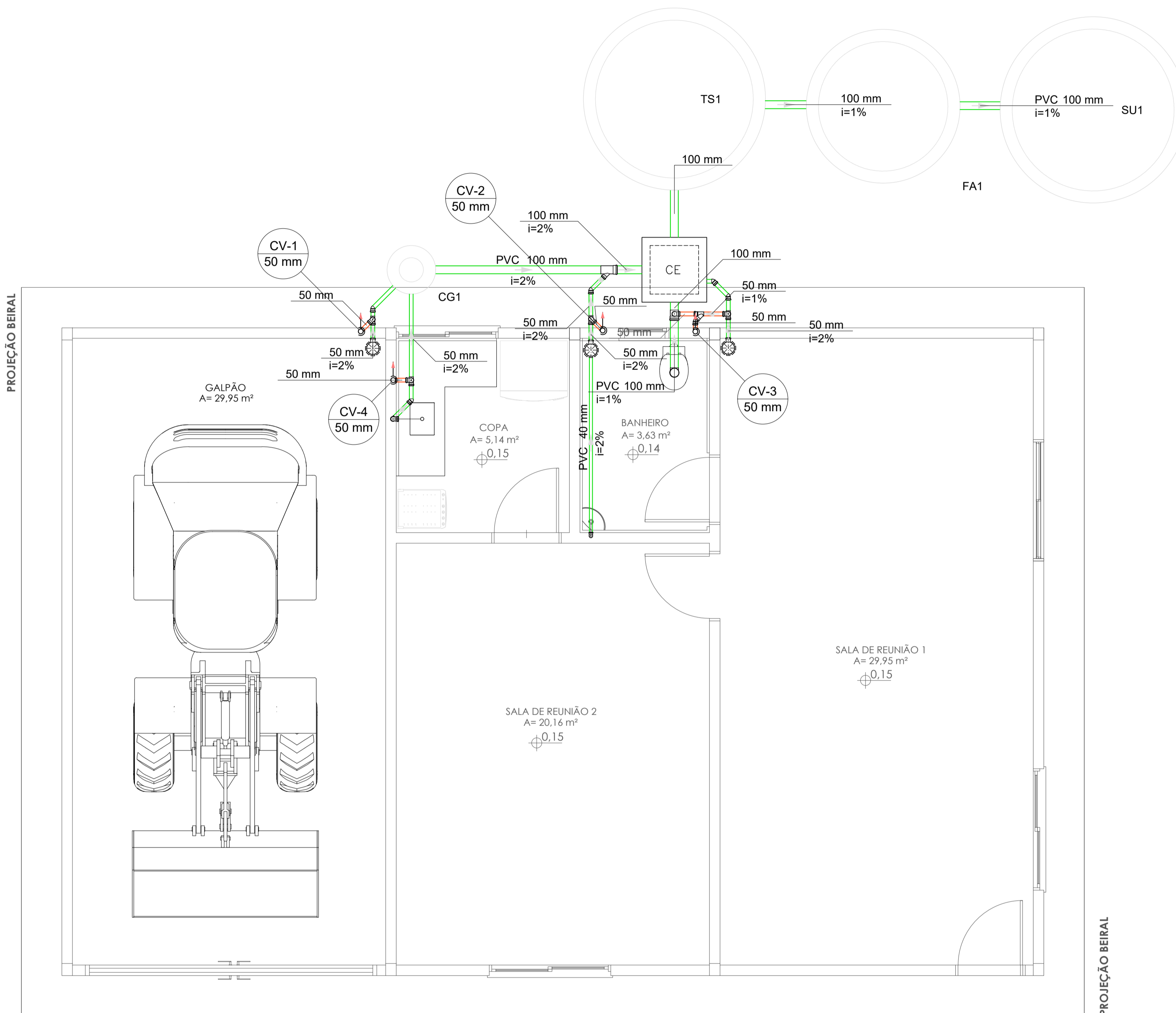
01 TÉRREO - SANITÁRIO ESCALA 1:75
